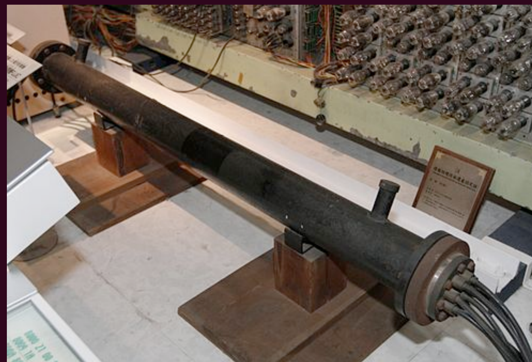
延迟线：实现存储器
