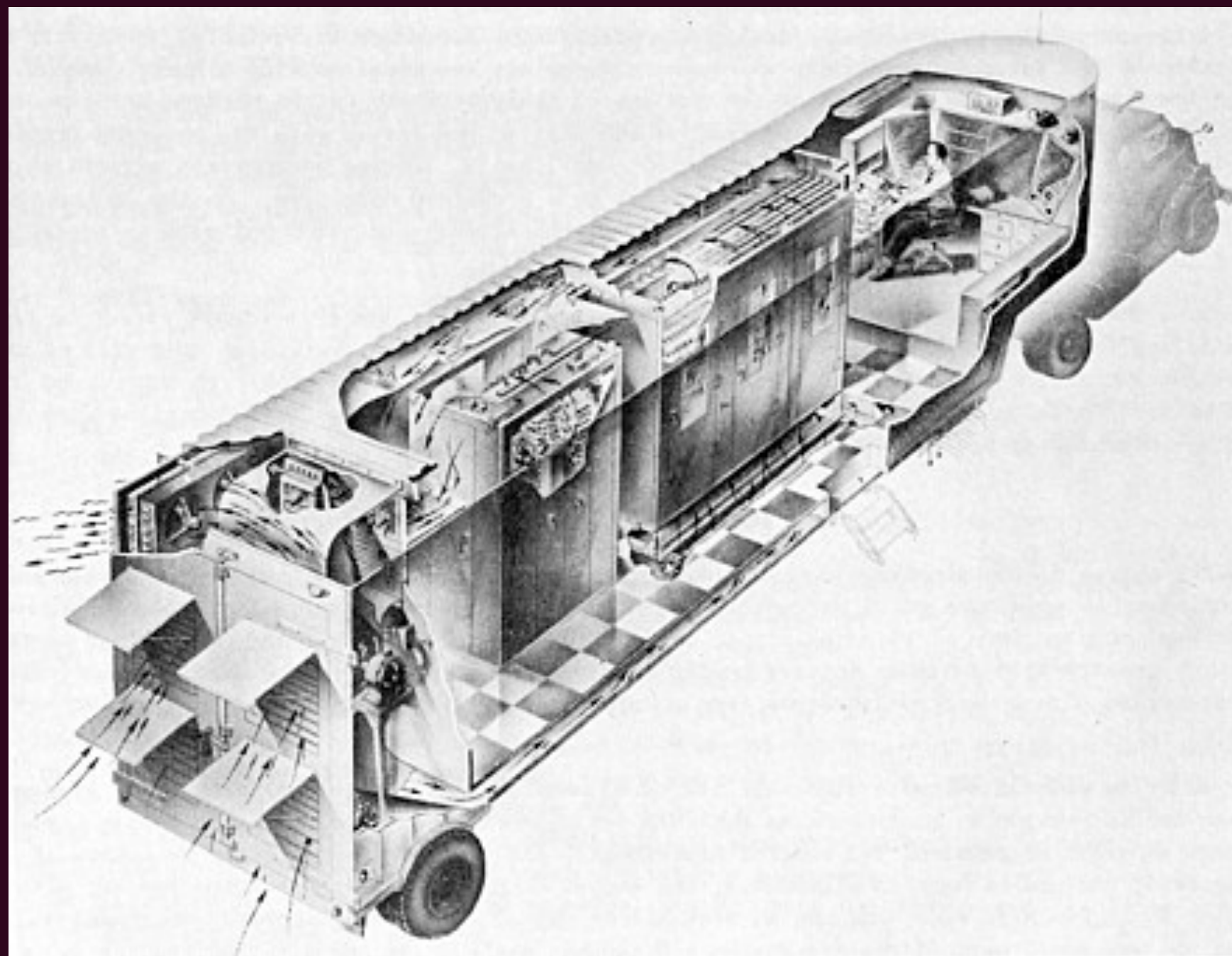
DYSEAC: 第一个使用中断的计算机，建在一个卡车里面
